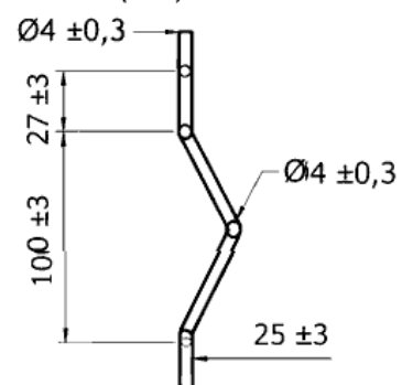
DETAL B (1:2)
