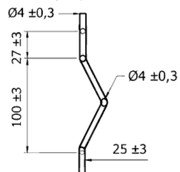
DETAL B (1:2)
